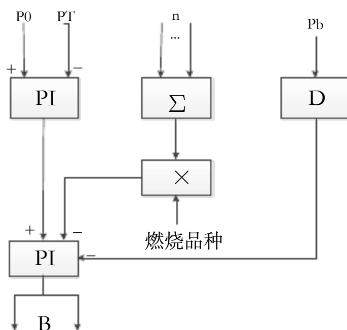
图 3.燃料量控制系统
