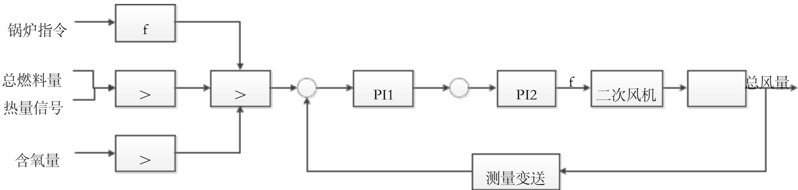
风量控制方框图
