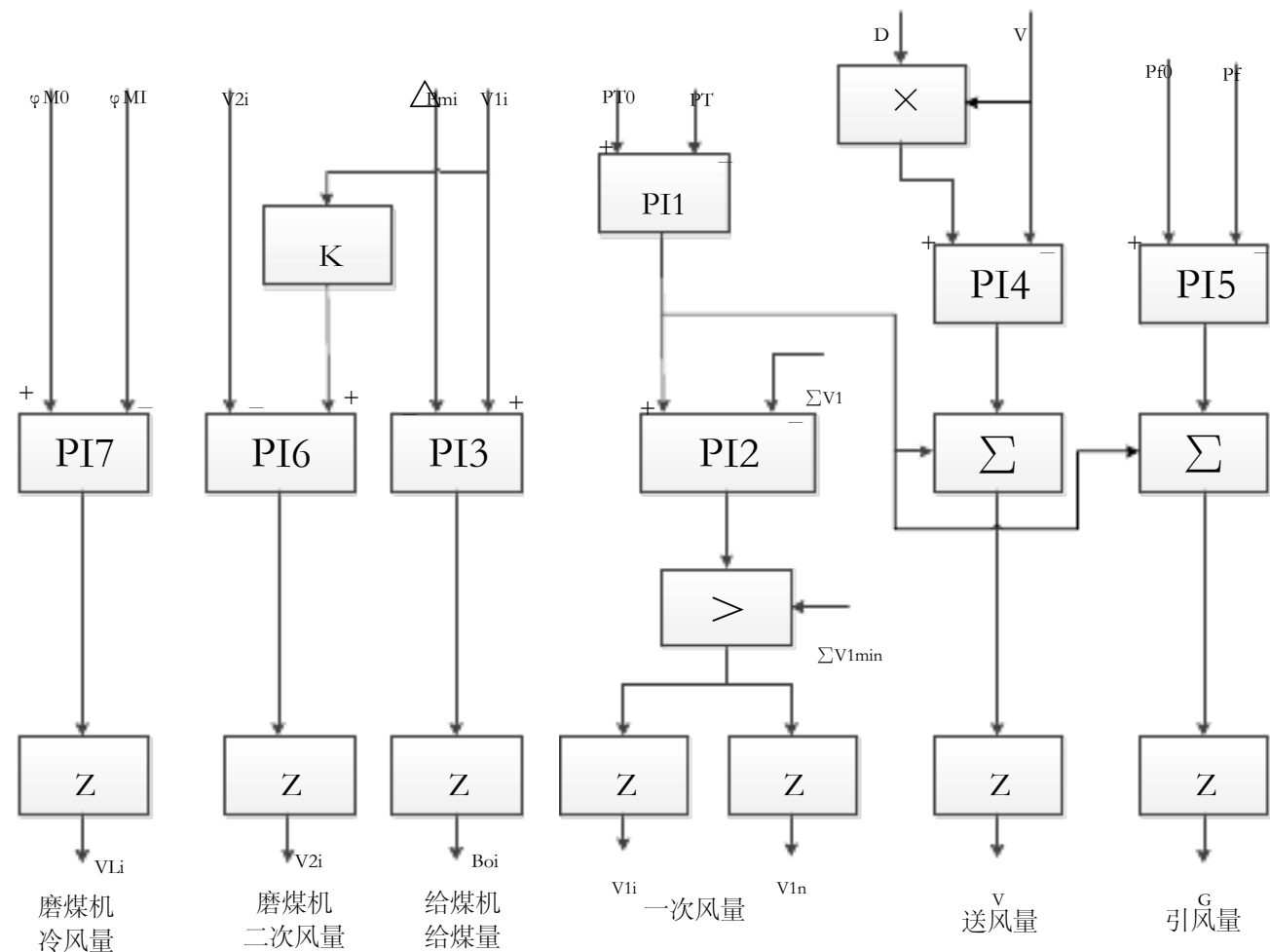
图 5. 一次风量为反馈信号的燃烧控制系统
