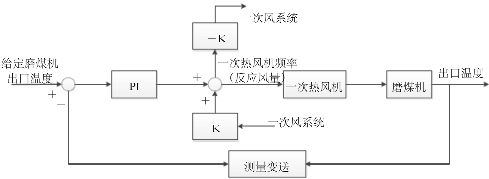
机出口温度控制方框图
