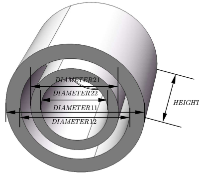
图 2 线圈结构图
