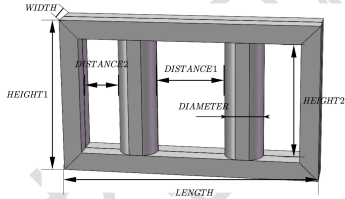
图 1 双心柱有旁轭结构图
