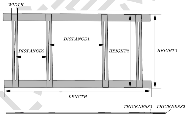
图 3 夹紧件结构图
