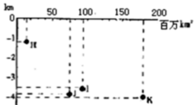
乙 四大洋 (H-K) 面积和平均深度示意图
