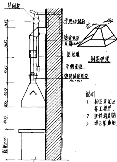
侧面
