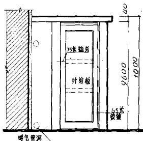
立面
