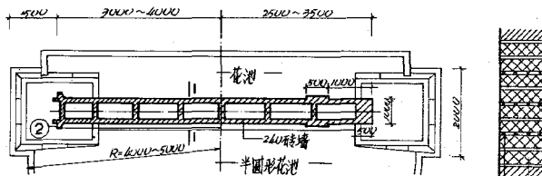
平面
