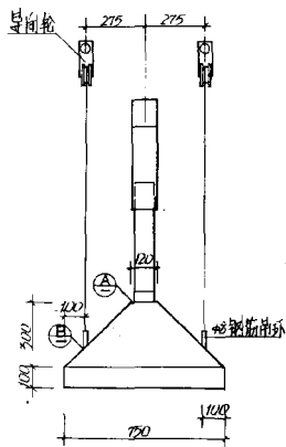
立面
