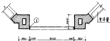
平面
