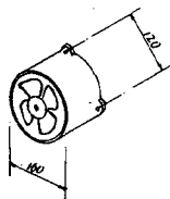
排风机
