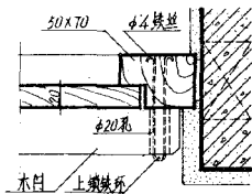
① 木框固定展览板
