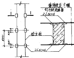
剖面
