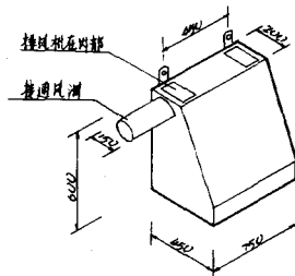
轴侧图
