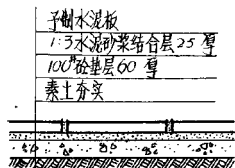
庭园地坪①③做法
