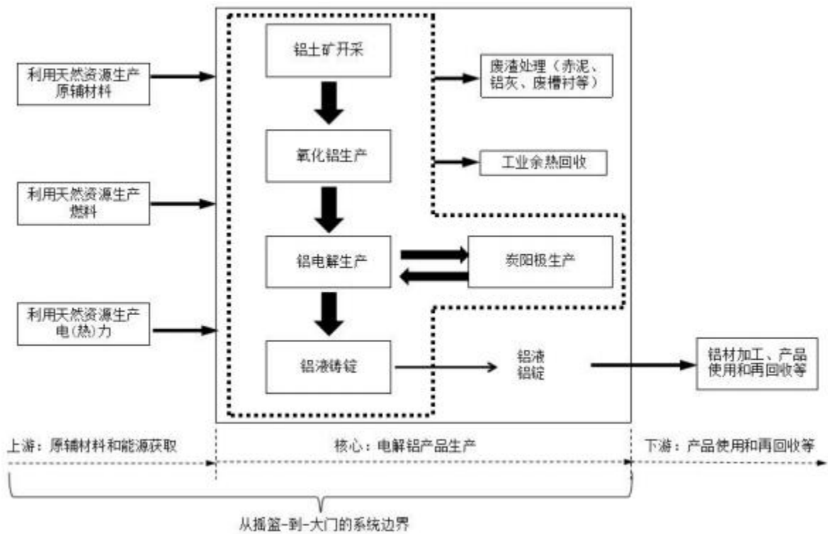
图 1 电解铝产品生命周期系统边界图
