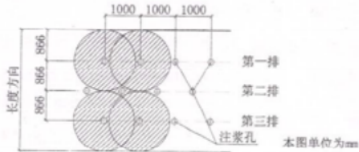
图<T3-3.2.4-01> 双液分层注浆布孔示意图
