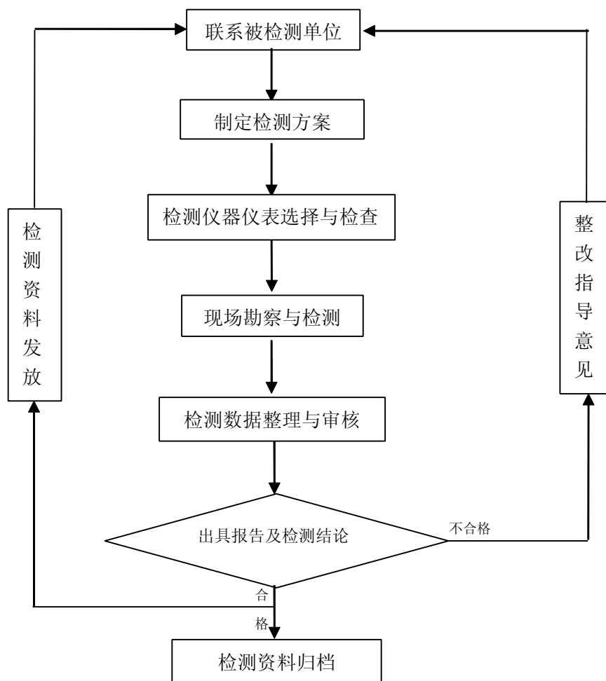
图1 电子信息系统防雷检测流程图
