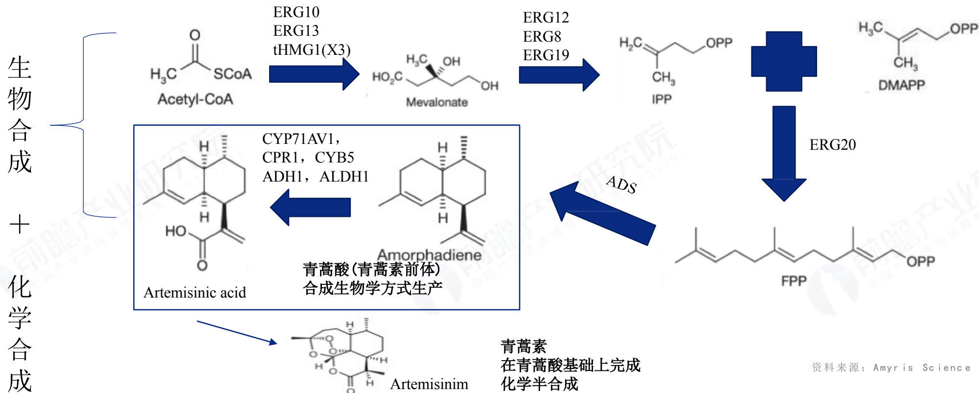
Amyris规模化生产青蒿素生物合成与化学合成结合办法
