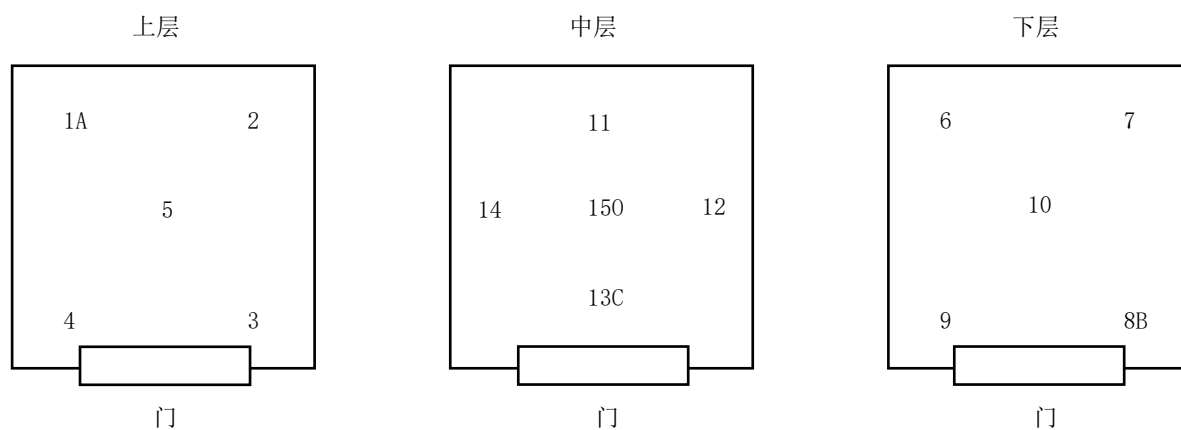
图 4 试验箱容积大于 2\text{ m}^3 布点示意图
