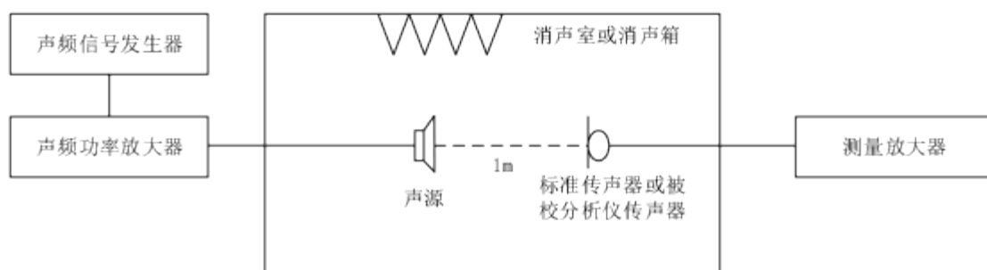
图 2 频率计权 (A 计权) 校准原理框图
