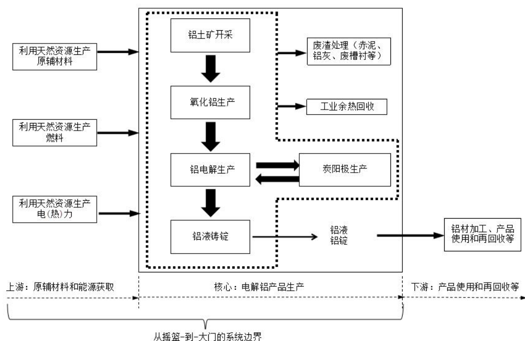
图1 电解铝产品生命周期系统边界图
