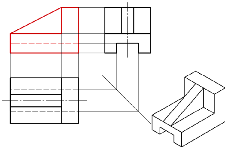
3-6-3 补画主视图 (保留投影连线)。
