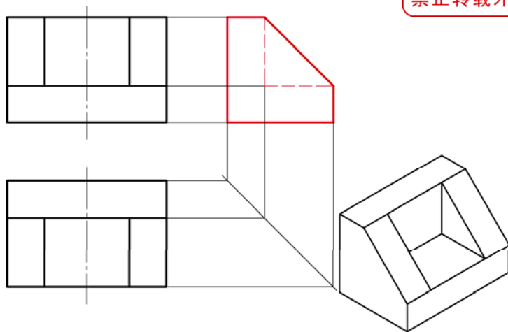
3-6-4 补画左视图 (保留投影连线)。
