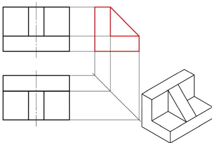
3-6-4 补画左视图 (保留投影连线)。
