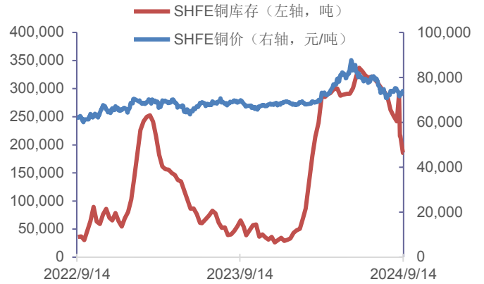
图 14 : SHFE 铜价及库存
