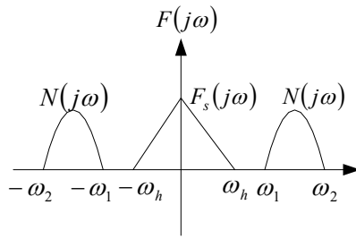
图2-14 信号频谱图
