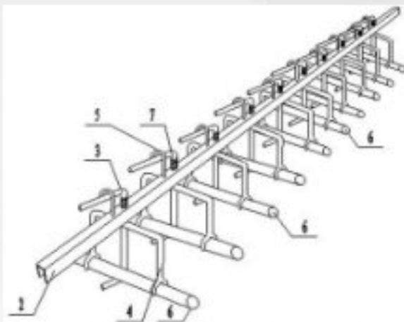
图3-1 一种混凝土铺面接缝传力杆定位支架
