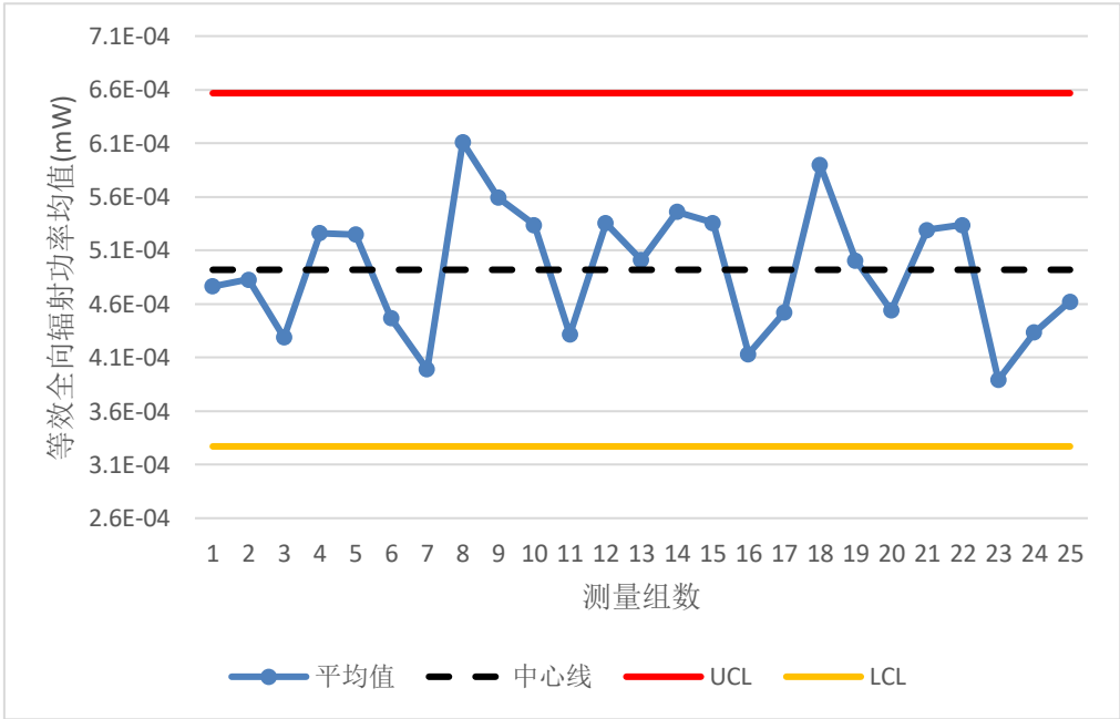
图 A.2.2 初始均值 \bar{X} 图
