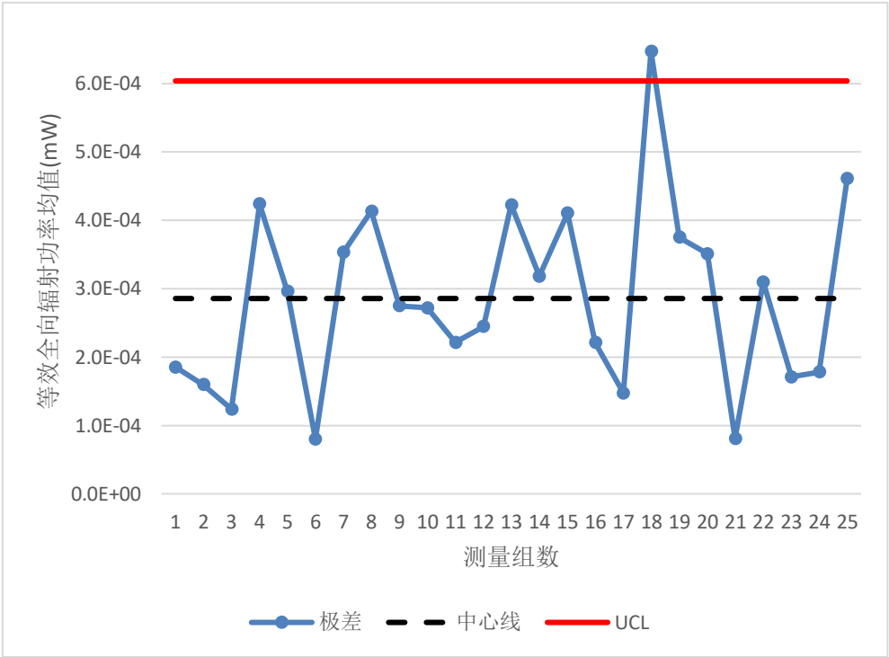
图 A.2.1 初始极差 R 图
