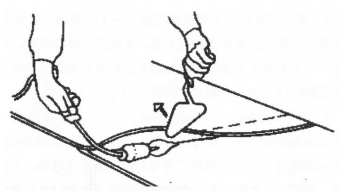
图 1 搭接缝熔焊粘结示意图
