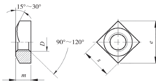
图 1 方螺母的型式
