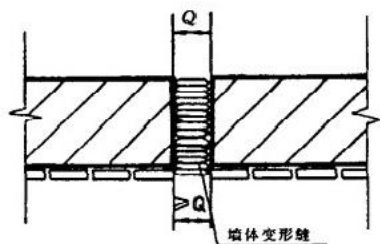
图4.0.6 变形缝两侧排砖示意
