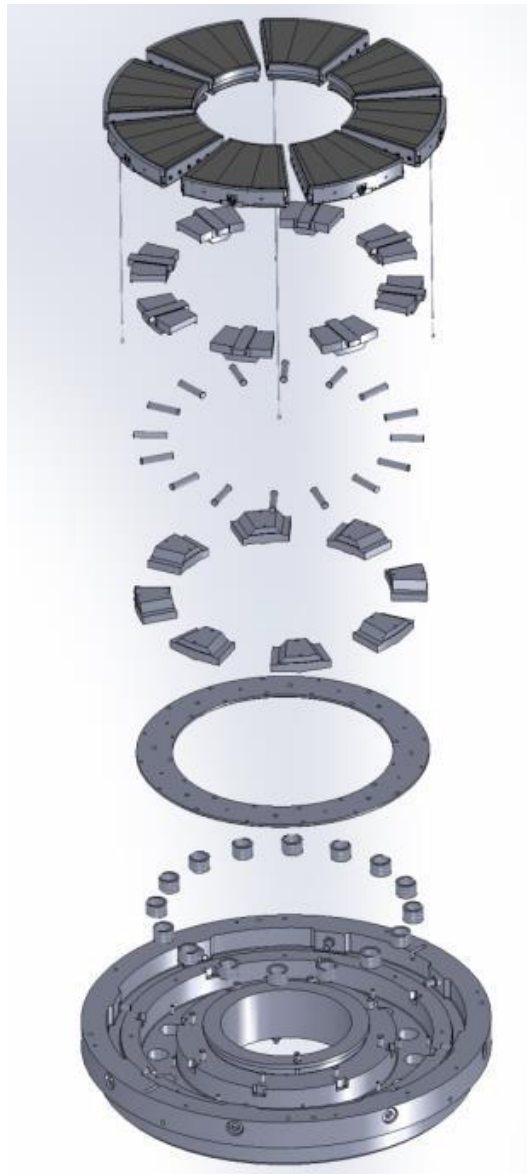
图 1 水润滑推力轴承爆炸图
