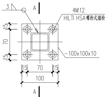
埋铁大样图
