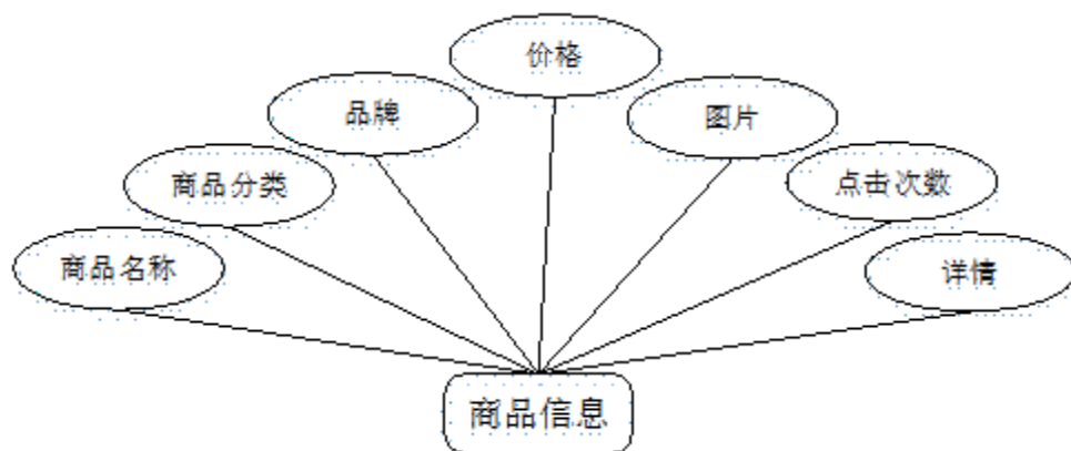
图 4-2 商品信息 E/R 图
