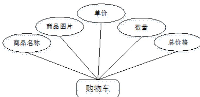
图 4-3 购物车 E/R 图
