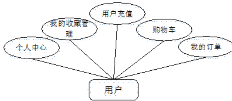
图 3-2 用户用例图
