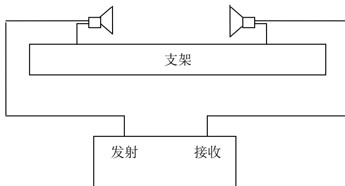
图2 平面测试换能器声时测量相对误差（声信号方法）的校准装置示意图
