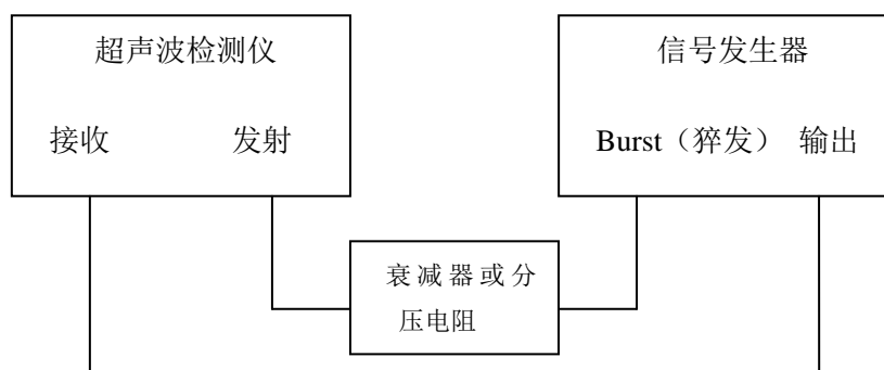
图 1 超声波检测仪声时测量（电信号方法）校准装置示意图
