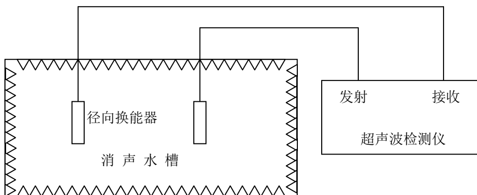
图3 圆管径向辐射换能器声时测量相对误差（声信号方法）的校准装置示意图
