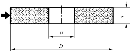
图 1 1 型砂轮
