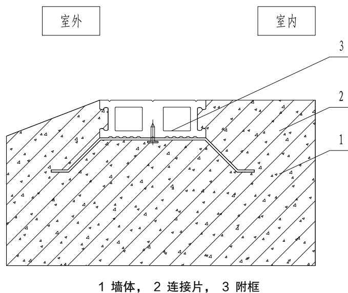
图 12 标准化附框前装式构造示意图
