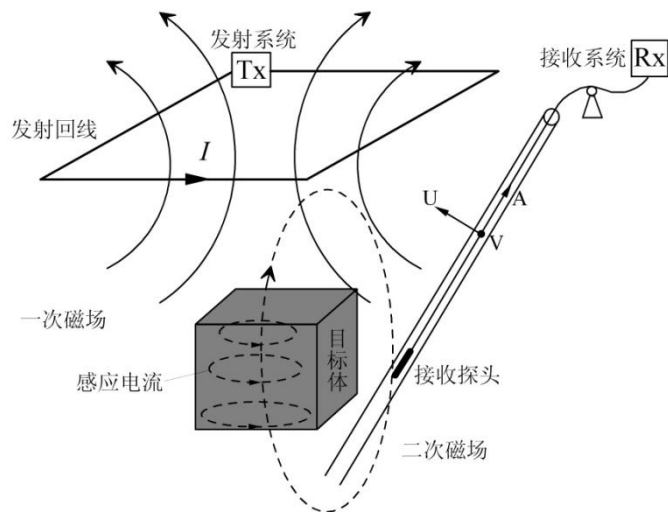
图1 地一井瞬变电磁法工作原理示意图
