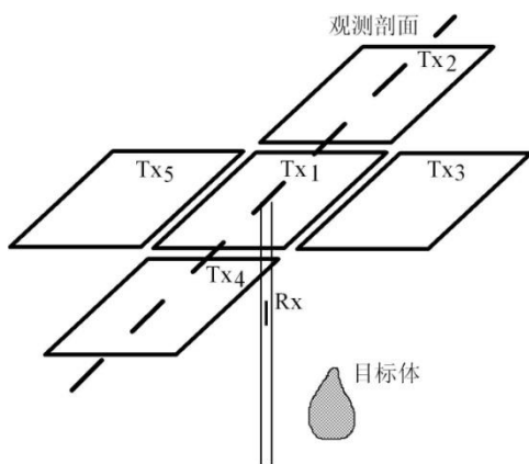
图2 五方位发送回线装置示意图
