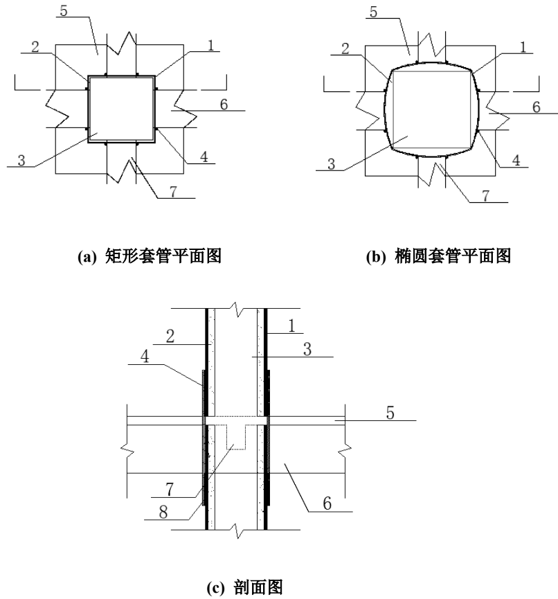
1-套管；2-后浇灌浆料；3-原钢筋混凝土柱；4-穿过楼板的钢筋或钢板条； 5-原楼板；6-原主梁；7-原次梁；8-焊缝
