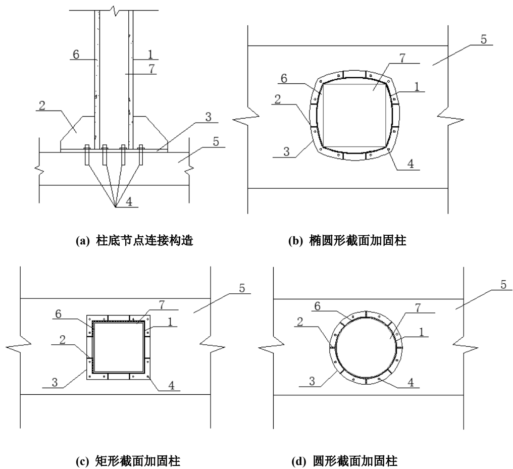
1-加固柱；2-加劲肋；3-对焊的钢制环形底板；4-扩孔自锁锚杆； 5-基础；6-后浇灌浆料；7-原钢筋混凝土柱
