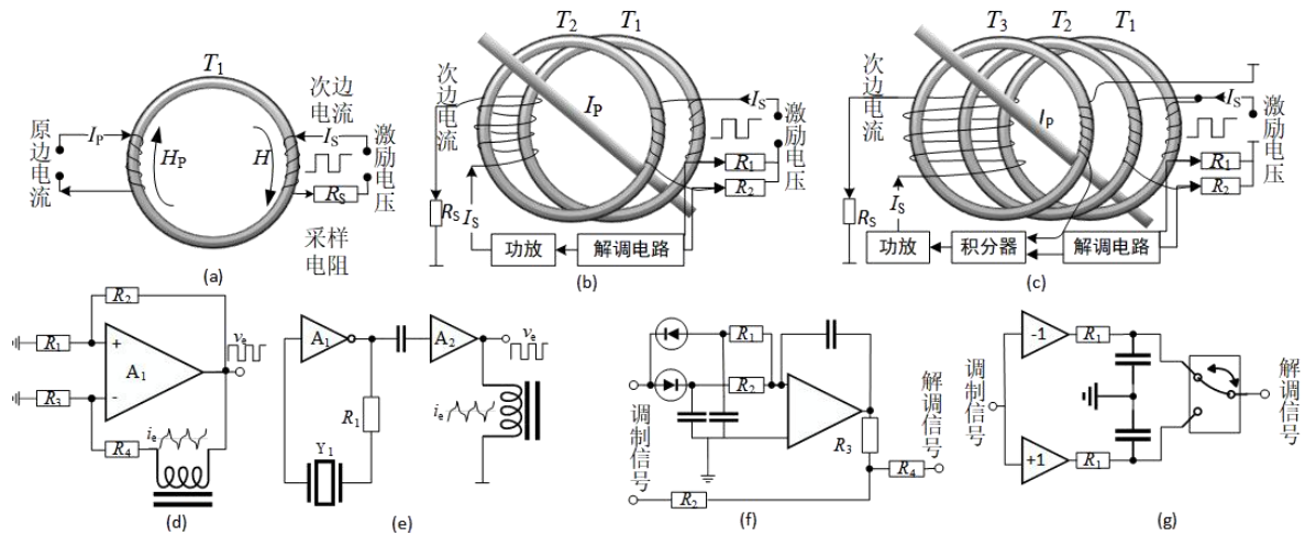
图1 磁通门电流传感器结构及原理
