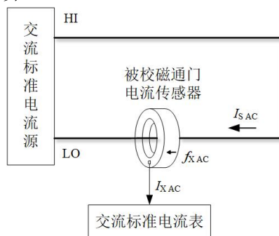
图 5 直接测量法的交流电流比例校准原理图
