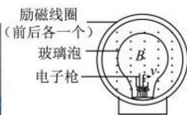
乙 结构图
