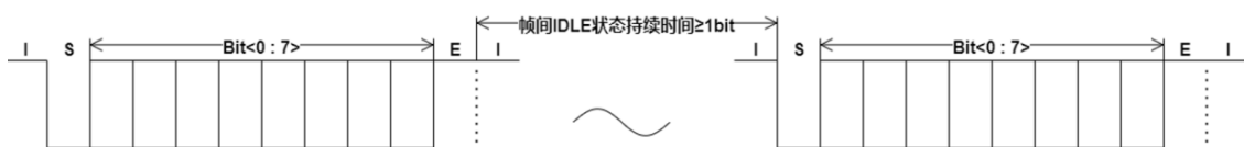
图7 数据帧间时序要求
