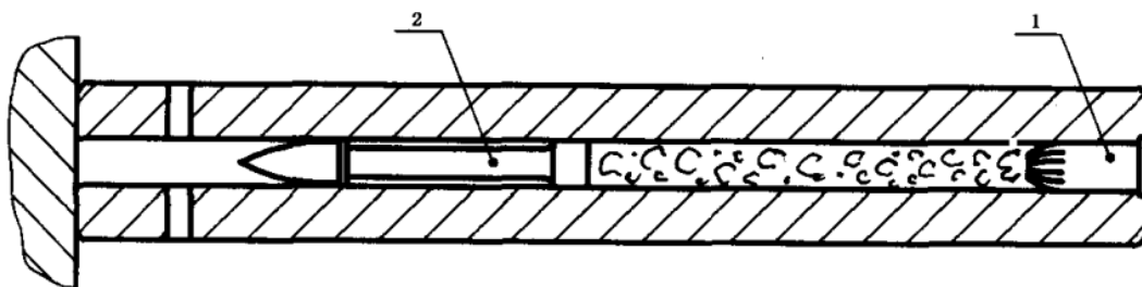
1—射钉弹； 2—射钉
