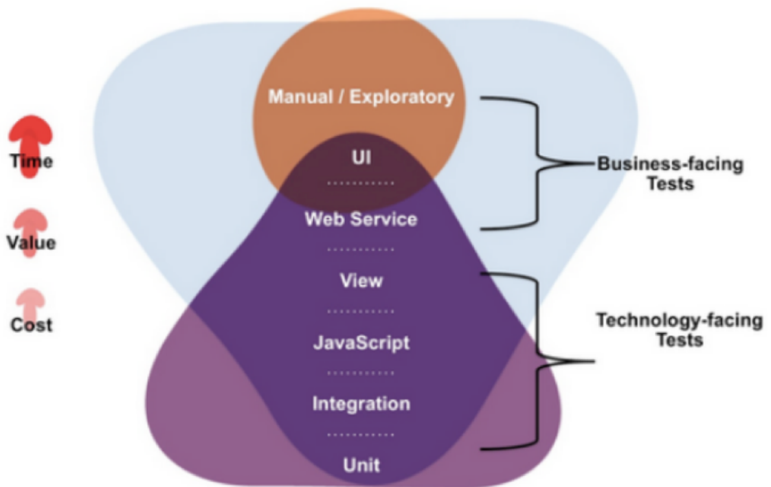
图1 测试金字塔
