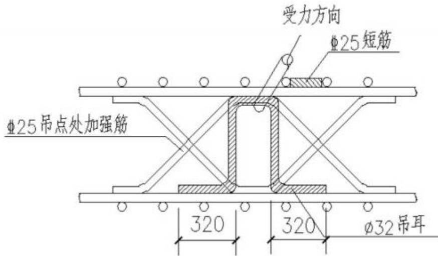
图 5.2.3-10 钢筋笼吊点大样图
