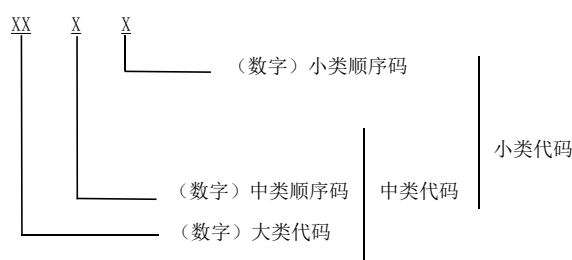
图2 代码结构
