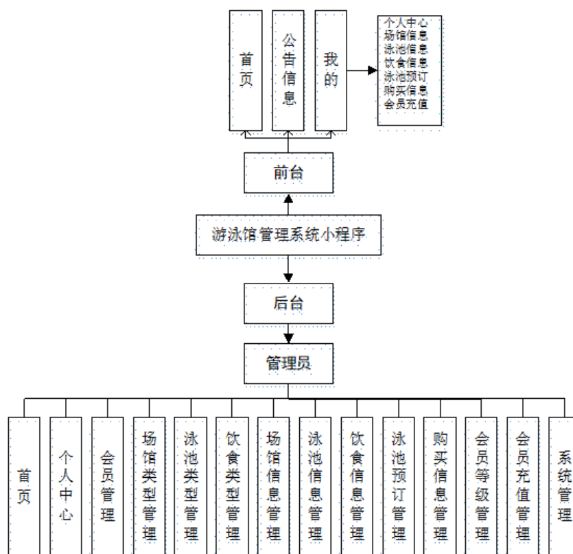
图 4-1 小程序总体功能模块图
