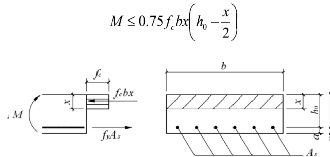
图 3 配筋受弯条板正截面承载力计算简图
