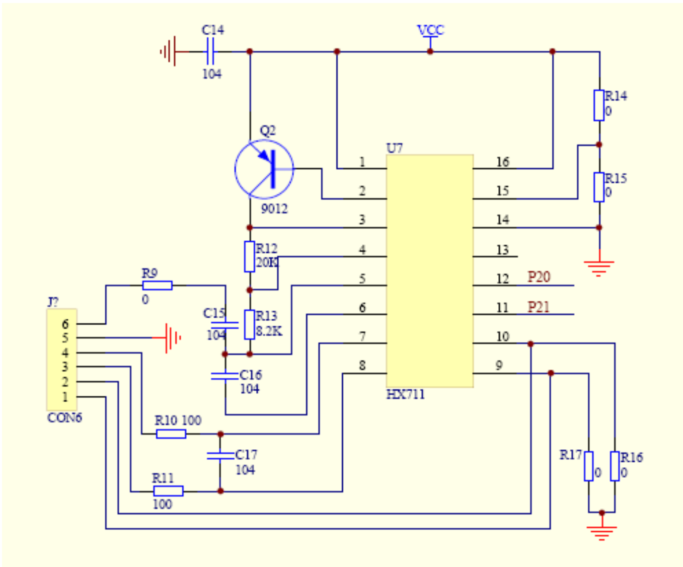
图 3.4 HX711 电路图
