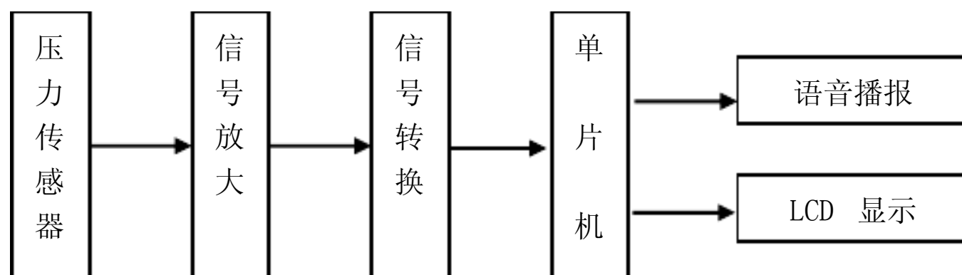
图 2.1 设计框图
