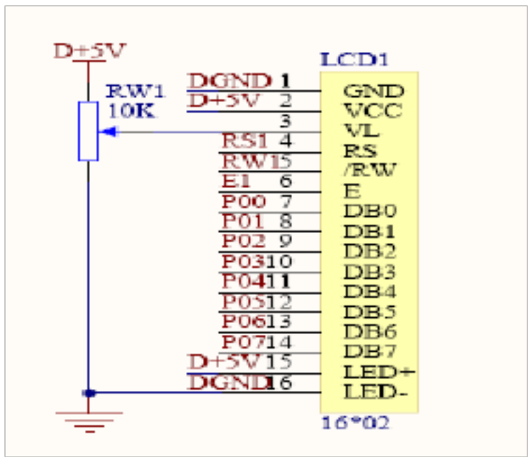
图 3.5 LCD1602 电路图
