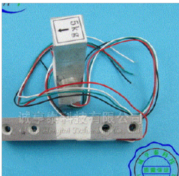
图 3.2 称重传感器
