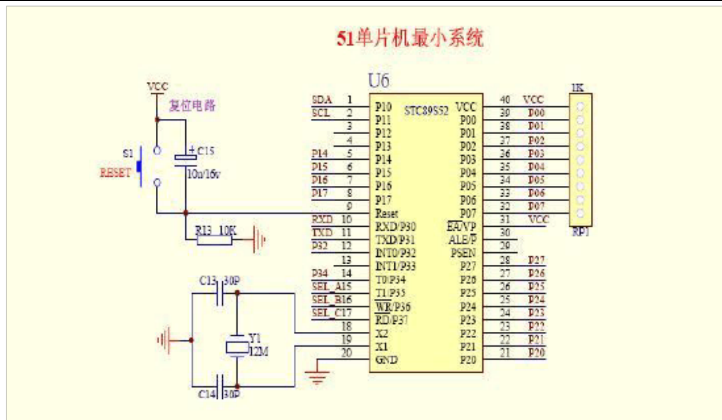
图 3.1 单片机电路
