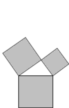
第一代勾股树
