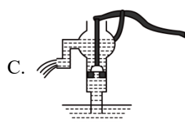
活塞式抽水机的手柄
