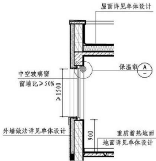
① 直接受益窗构造
