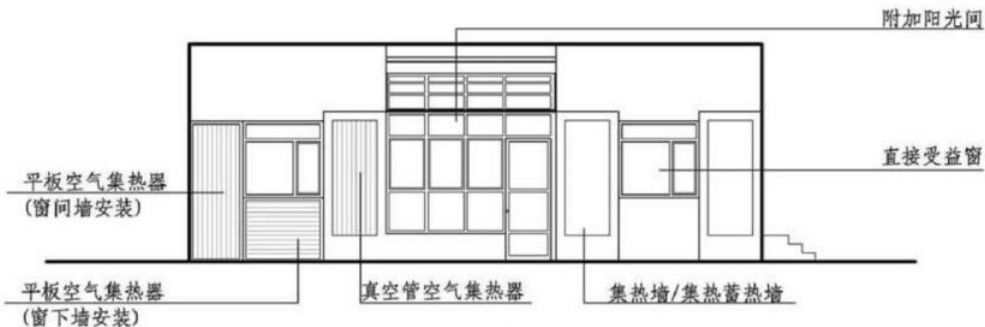
被动式太阳能采暖技术立面索引图
