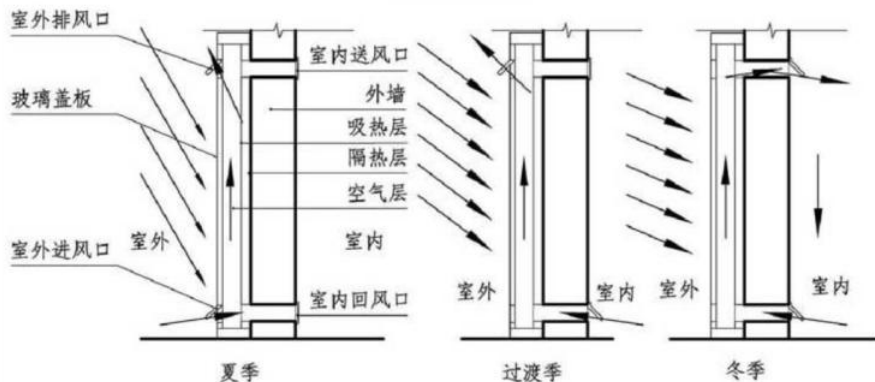
集热墙
