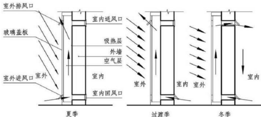
集热蓄热墙
