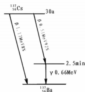
图 1-5 {}^{137}\text{Cs} 的 \beta 衰变纲图
