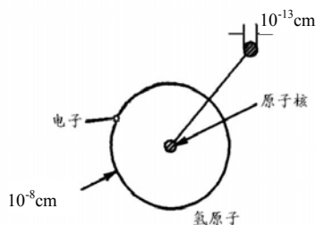
图 1-1 氢原子核结构示意图
