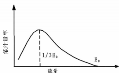
图 1-4 \beta^- 的粒子的能量分布曲线
