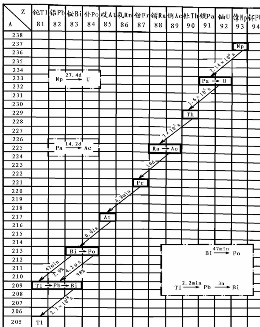
图1-12 镭系衰变图
