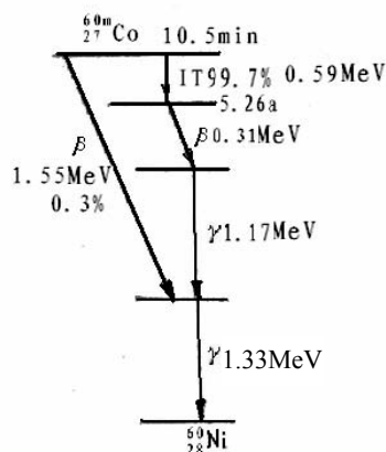
图 1-8 ^{60}\text{Co} 衰变纲图
