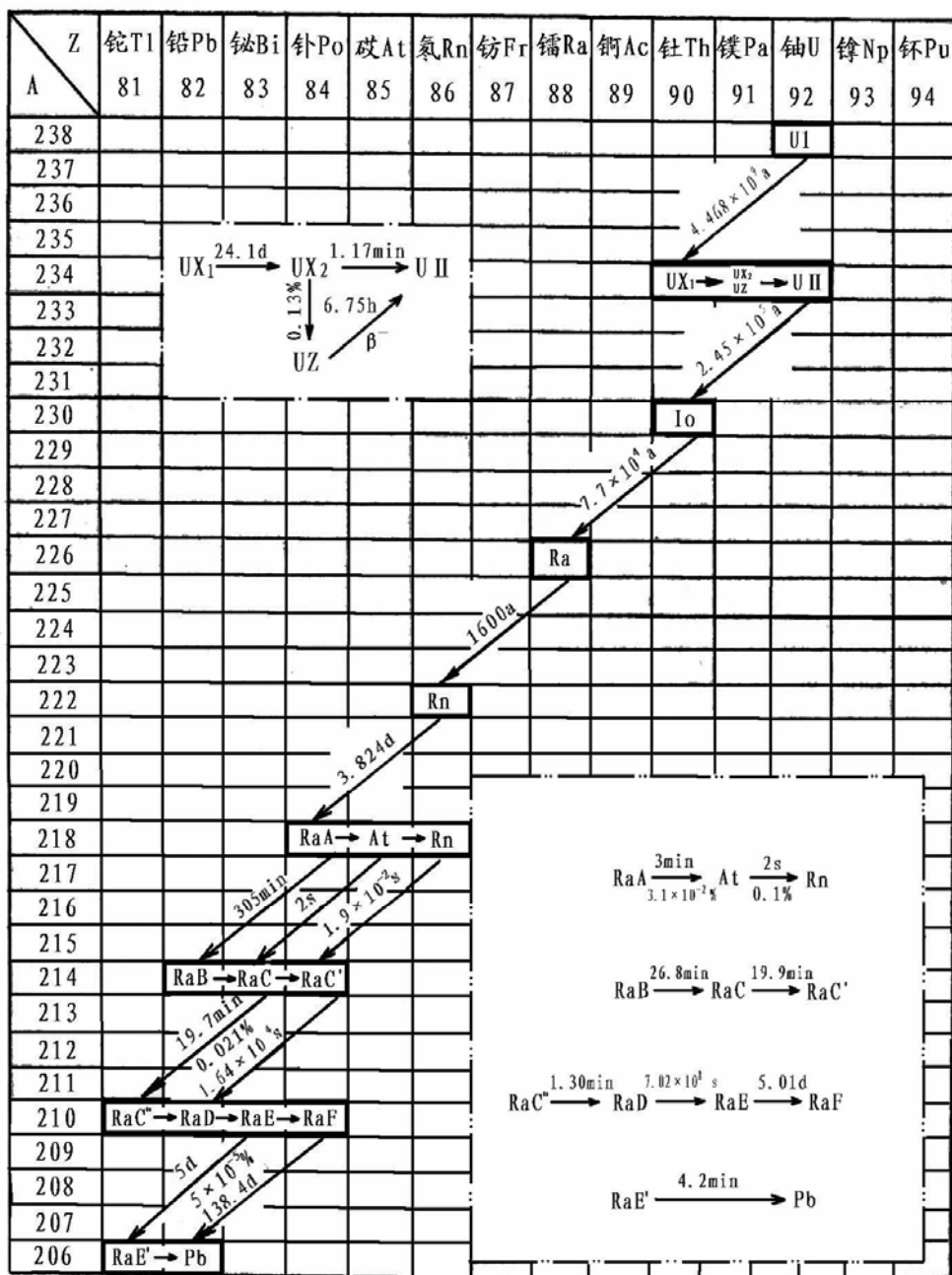
图 1-9 铀系衰变纲图
