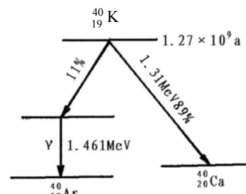
图 1-5 {}^{40}\text{K} 的衰变纲图
