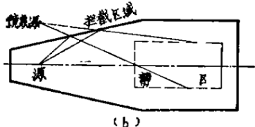
图1 微波暗室的工作情况。 (d) 在微波暗室轴上辐射源与镜象源距离均为 1/2 室宽。 (b) 由于锥形墙靠近源天线，镜象源也近了。
