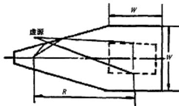
图 3 锥形暗室的尺寸选择
