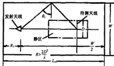
图 2 矩形暗室的尺寸选择
