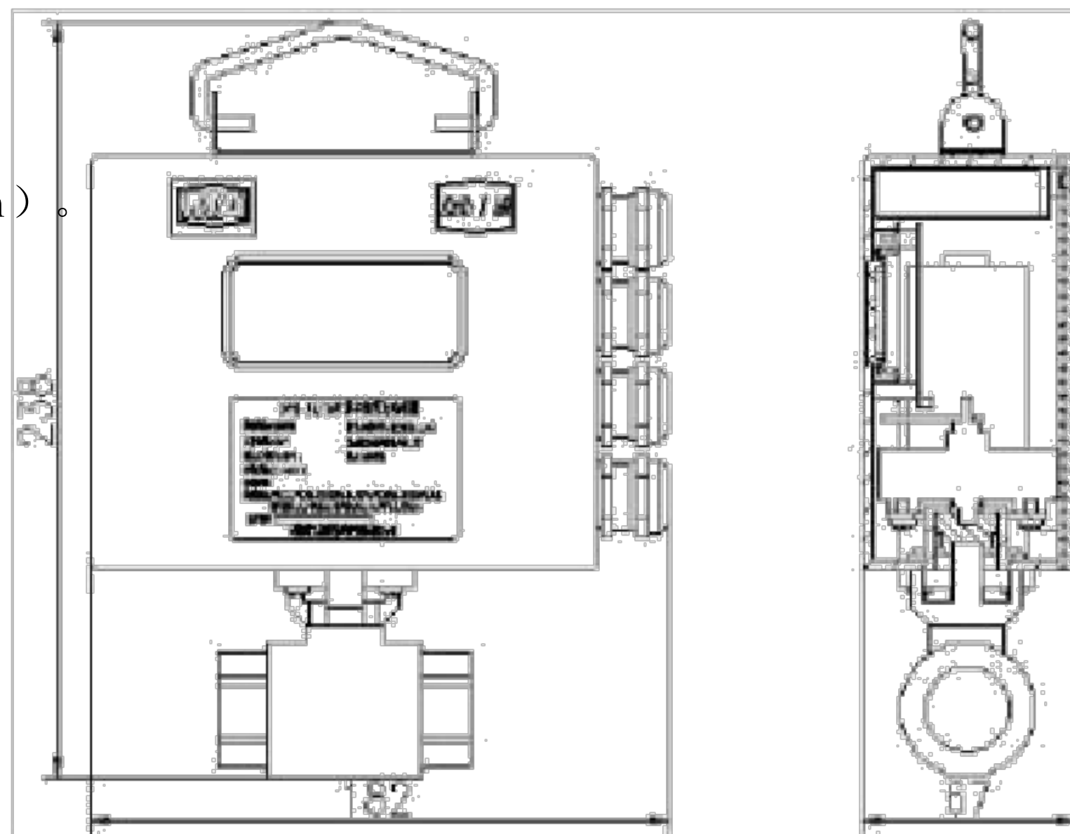
图 1 外形尺寸图
