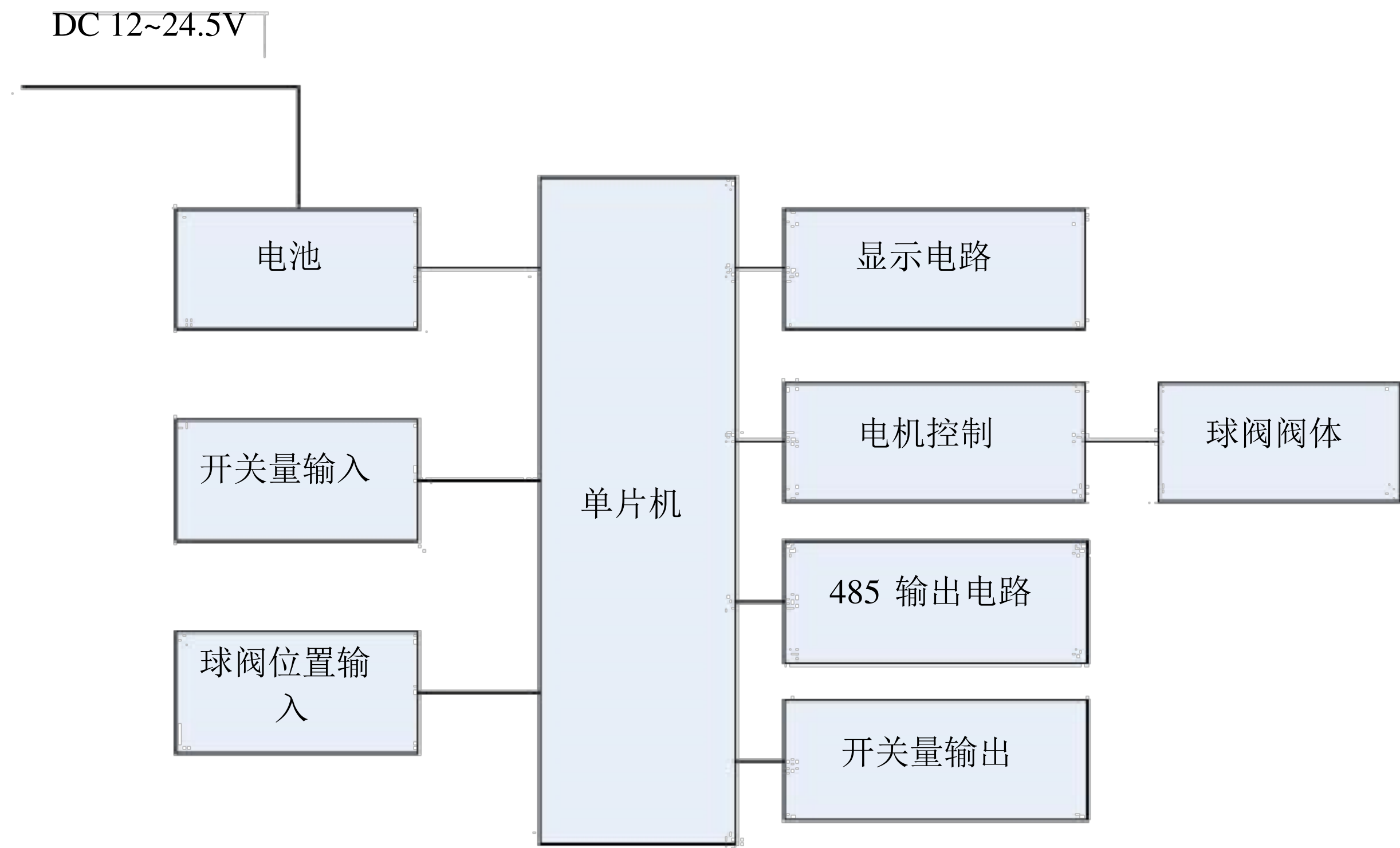
图 2. 电动球阀原理框图
