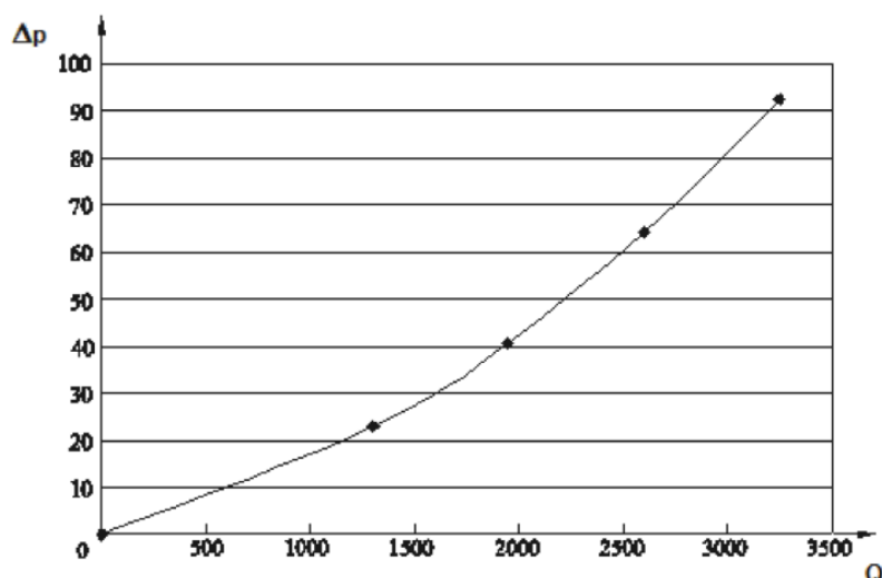
图 6 阻力随风量变化曲线示例
