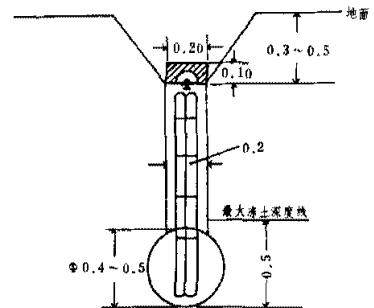
(f) 爆破型混凝土柱普通水准标石
