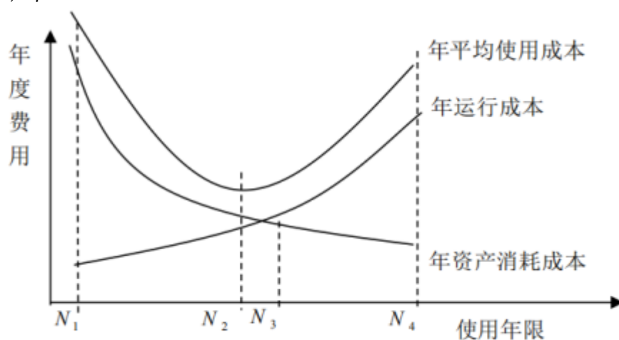
图 1 某设备年度费用曲线
