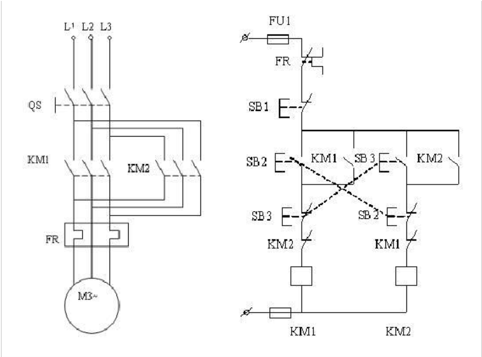
使用双重互锁，采用复合按钮和 2 个接触器。将 2 个接触器的常闭辅助触点相互串联在对方回路中，安全方便，避免了短路的发生~
