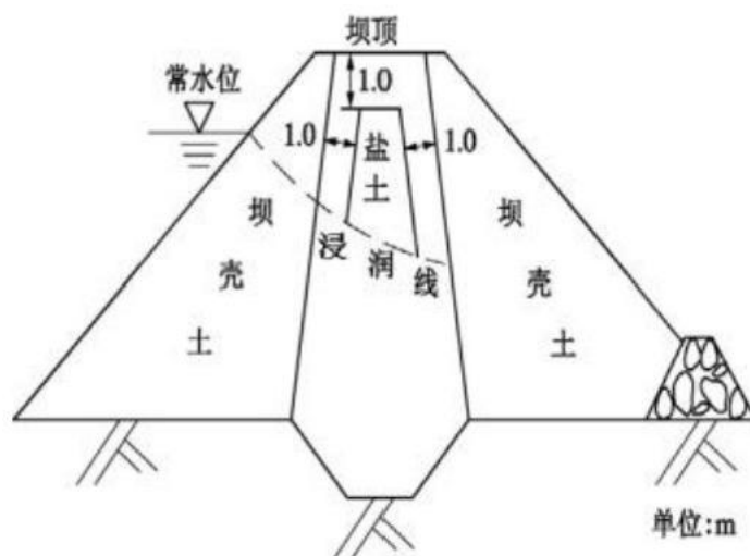
图B.2 心墙坝盐土铺垫位置断面图
