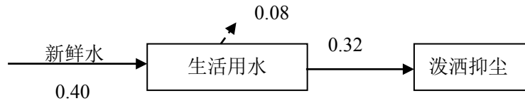
图1 水量平衡示意图 单位 (m 3 /d)
