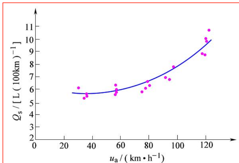
等速行驶百公里燃油消耗量曲线
