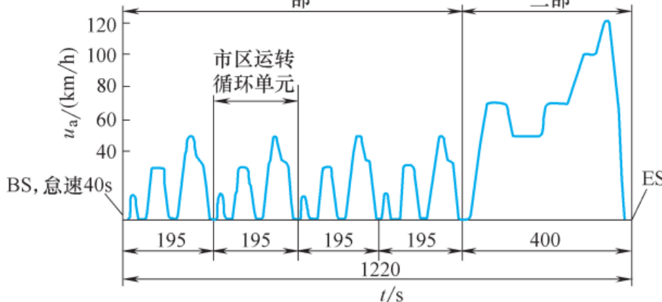
欧洲第二阶段油耗测试 车速-时间曲线
